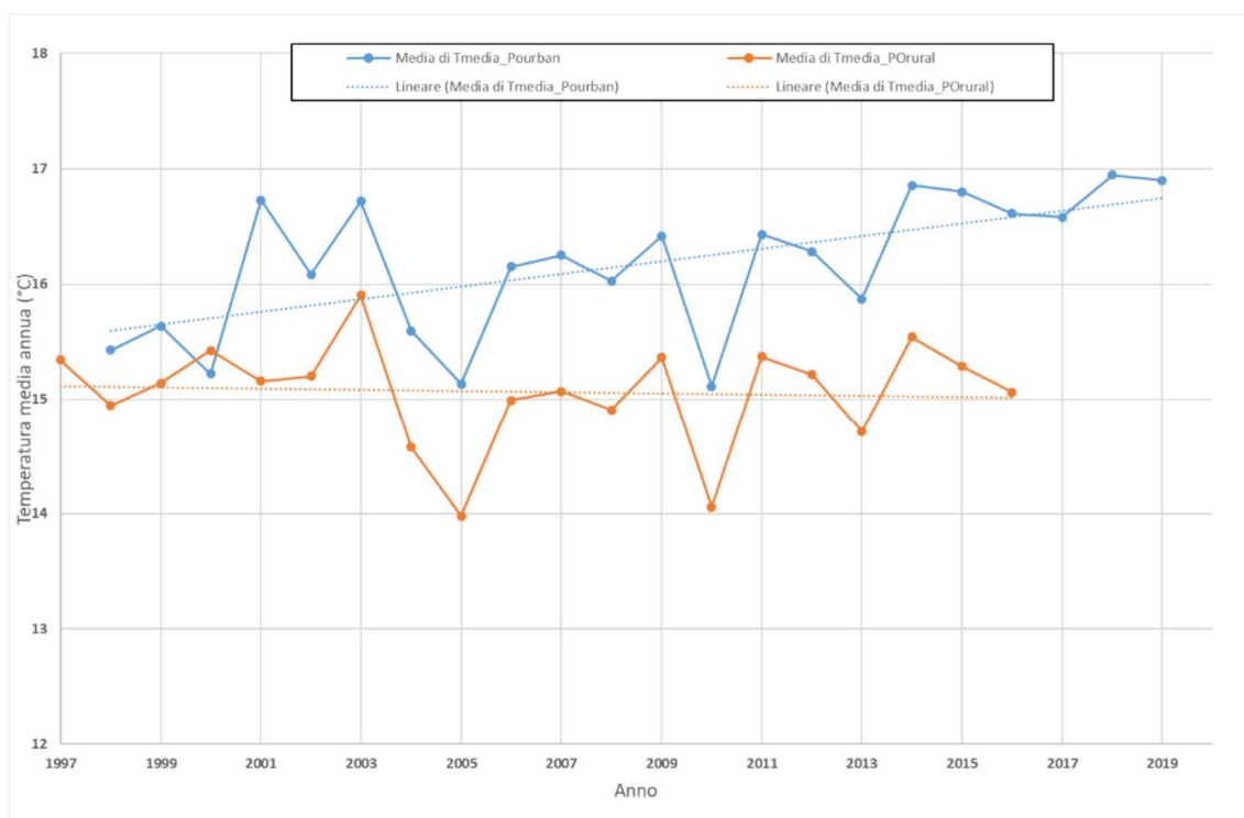
Figura 32. Andamento della temperatura media annua nel periodo 1997-2019
