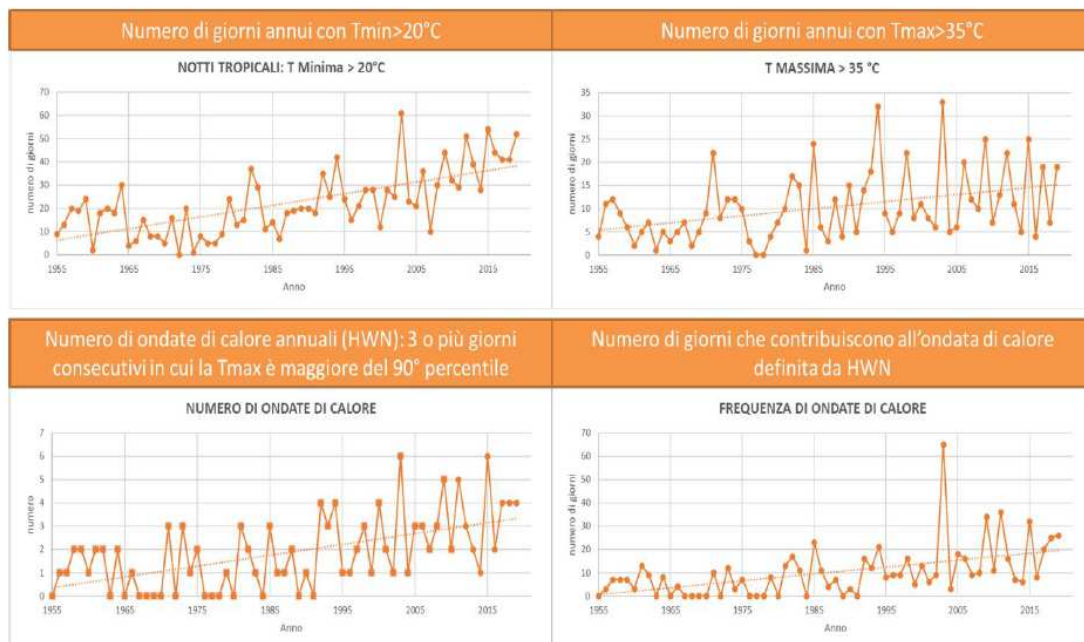
Figura 35. Andamento degli indici climatici notti tropicali, numero di giorni con temperatura massima > 35^{\circ}\text{C} , numero di ondate di calore annuale e frequenza delle ondate di calore dal 1955 al 2019 per la stazione Prato_Urban
