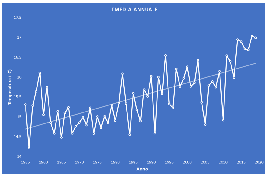
Figura 33. Temperatura media annua
