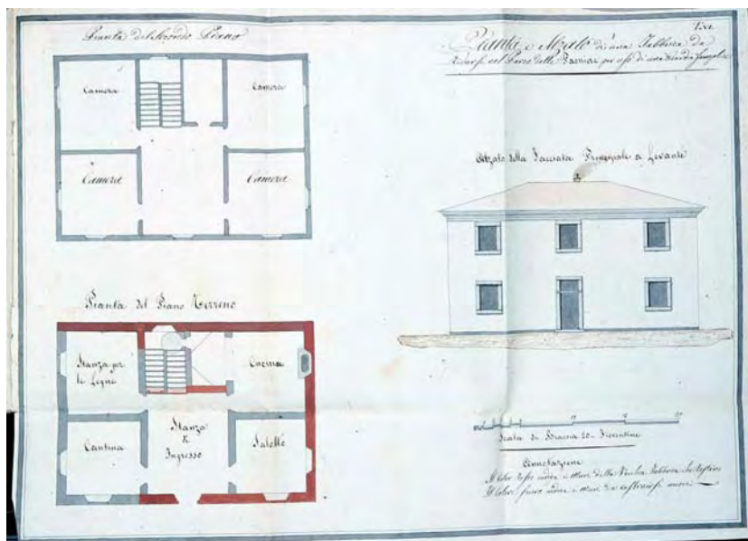
Casa per la guardia semplice Pianta prospetto e planimetria
