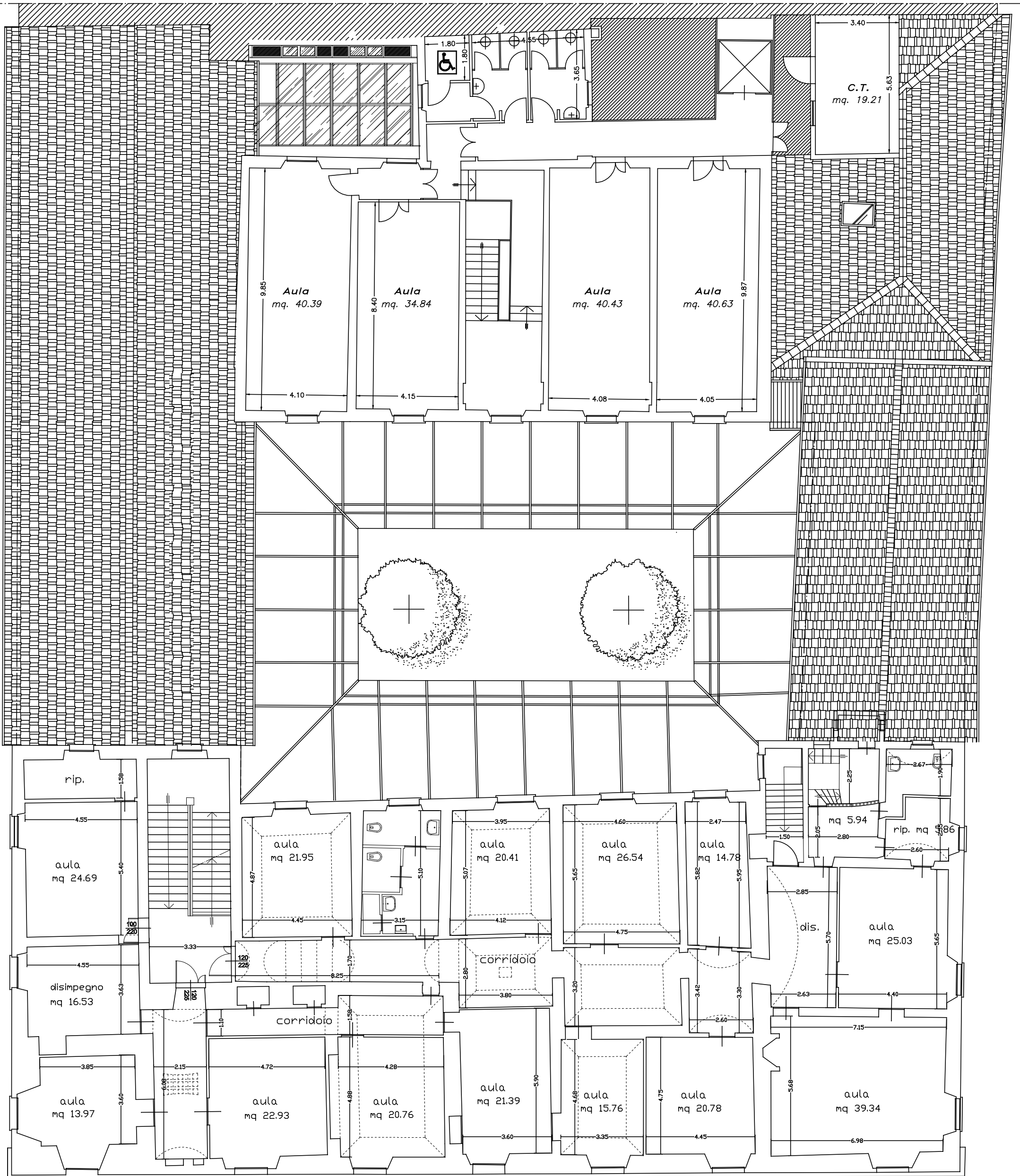
PIANTA PIANO SECONDO SCALA 1/100
